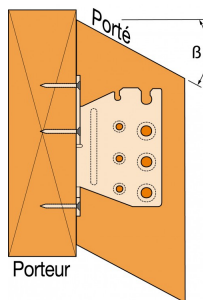
Anschluss mit Neigung an HT
